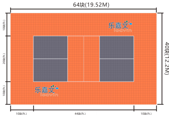
匹克球场地官方推荐尺寸
